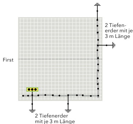
Variante 2: 4 x 3 m Tiefenerder
