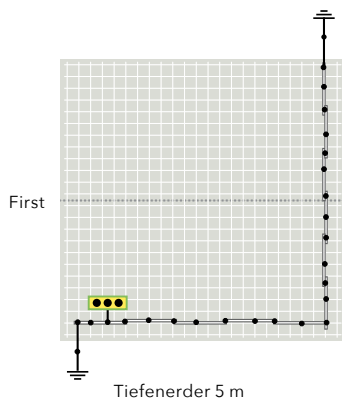
Variante 1: 2 x 5 m Tiefenerder
