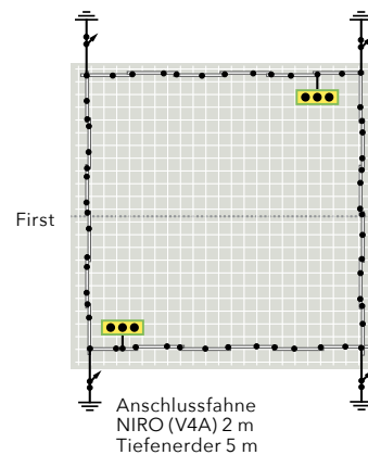
Variante 3: 4 x 5 m Tiefenerder (2 Erdungssets)
