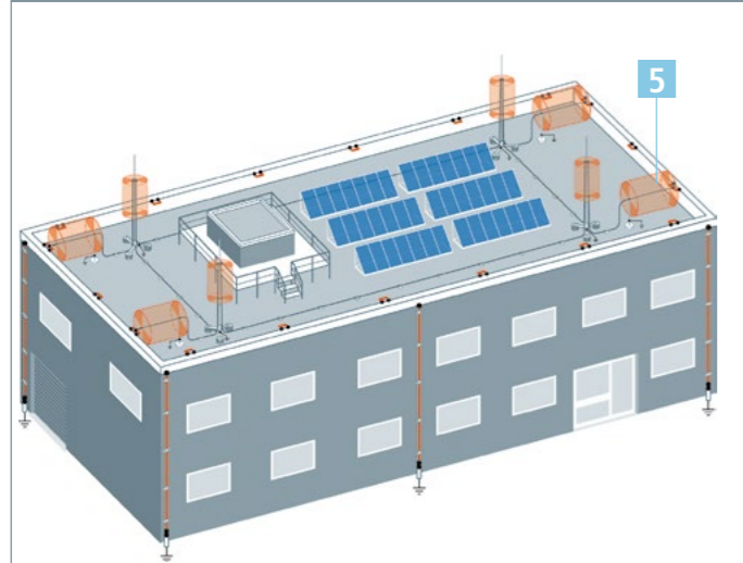
Getrenntes Blitzschutzsystem eines Verwaltungsgebäudes
