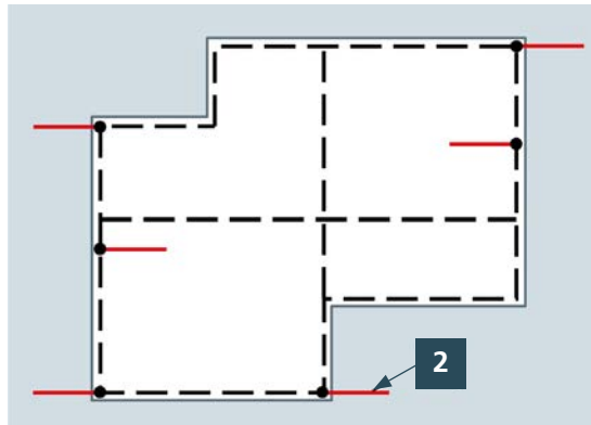
Erdungsfestpunkt Art.-Nr. 478 112
