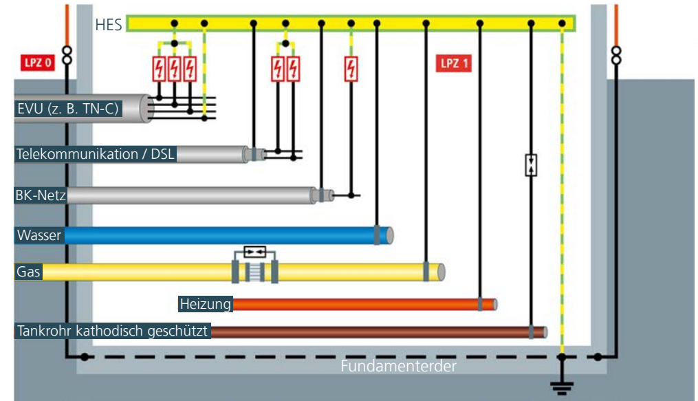
HES: Haupterdungsschiene, EVU: Energieversorgungsunternehmen, BK: Breitbandkabel (z.B. Kabel-TV)
