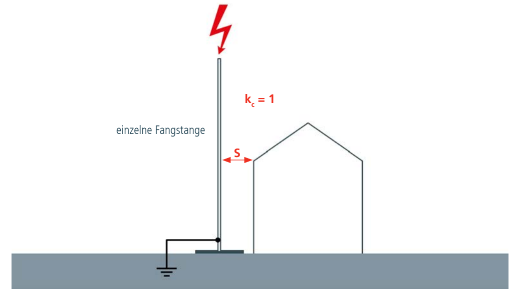
Trennungsabstand (s) / Zu leitfähigen und fremden leitfähigen Teilen
