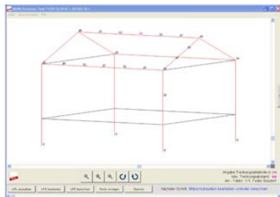
LPS III: Berechnung s für alle möglichen Einschläge
