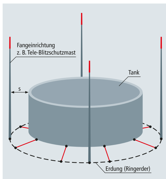
Bild 2 Fangeinrichtung für einen Tank mit Fangstangen und Fangseilen
