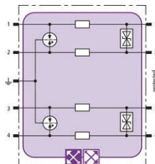
Prinzipschaltbild BXT ML4 BD HF 5
