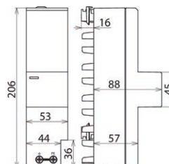
Maßbild DSH ZP TT 255
