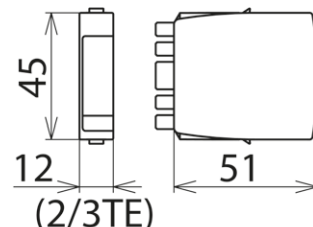
Maßbild BXT ML4 BD HF 5
