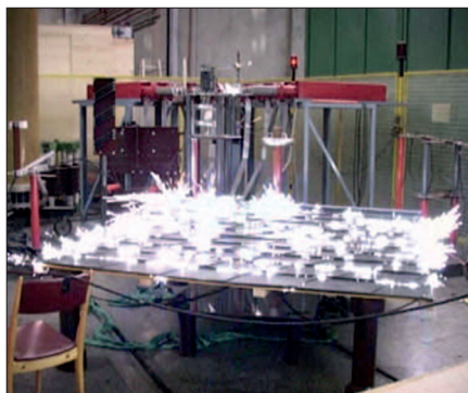
Obr. 4. Jiskření bleskového proudu na plechové střeše
