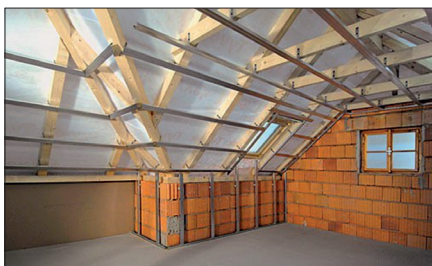
Obr. 1. Sádrokartonové profily v podkroví RD
