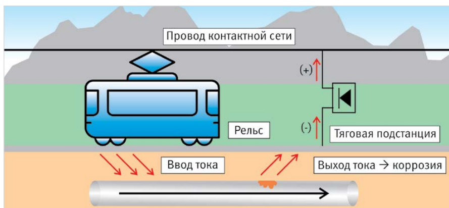
Рис. 2 — Протекание блуждающих токов, вызванных работой контактных сетей электрифицированного транспорта, по проложенному в земле трубопроводу
