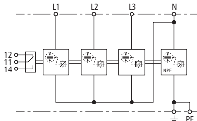
schemat połączeń DVA EMOB 3P 255 FM
