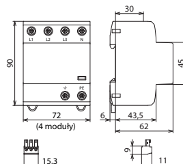
rysunek wymiarowy DVA EMOB 3P 255 FM
