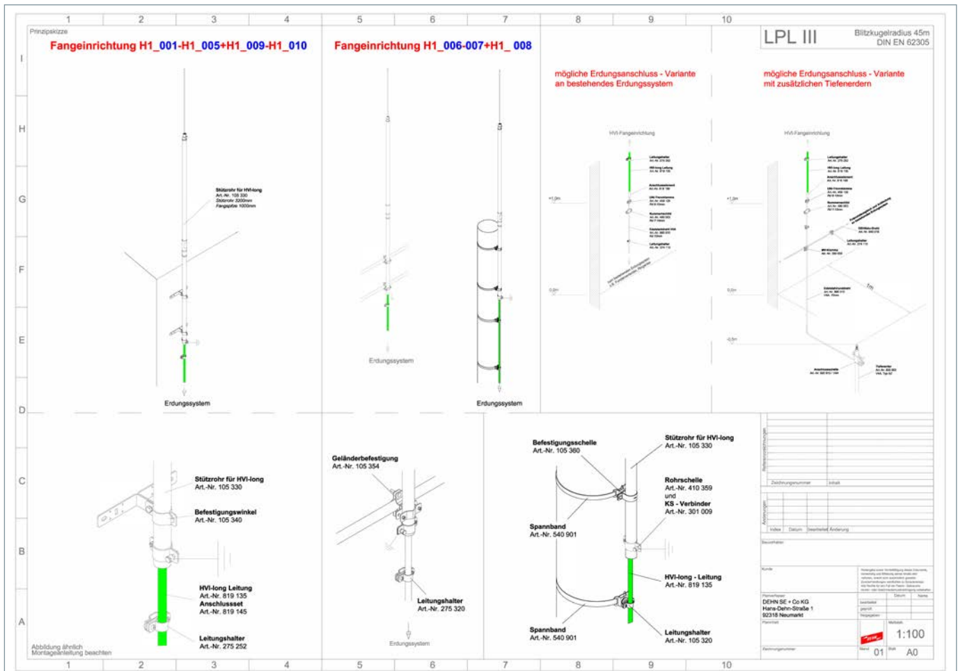
Detailsicht Blitzschutz
