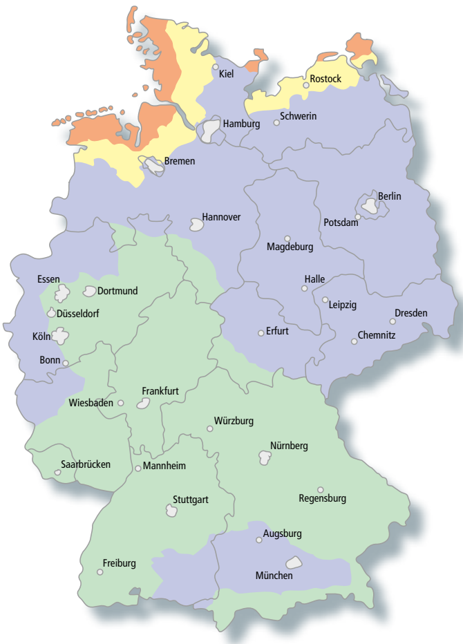
Bild 1: Windzonen in Deutschland
