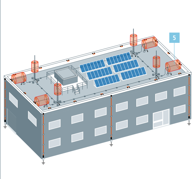
Getrenntes Blitzschutzsystem eines Verwaltungsgebäudes
