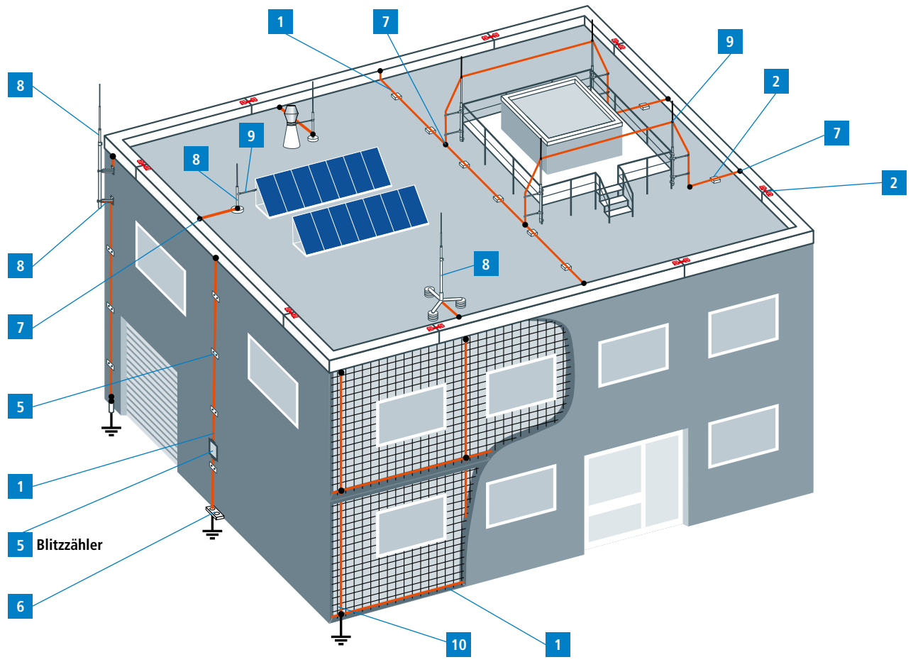
Äußerer Blitzschutz eines Industriegebäudes
