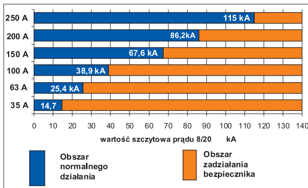
Rys. 4. Oddziaływanie prądu udarowego 8/20 na bezpieczniki
